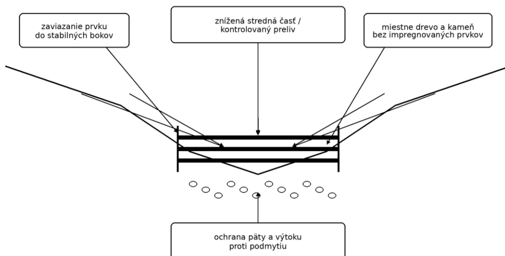
Obrázok 6.5 Schematický priečný profil malého dreveno-kamenného prehradzovacieho prvku pre drobnú eróznú dráhu. Zdroj: Vlastné spracovanie.
